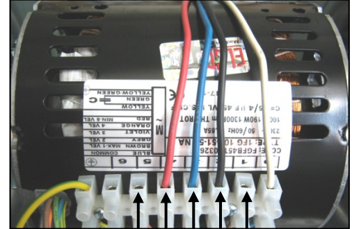
motor tapping: 5 4 3 2 1
