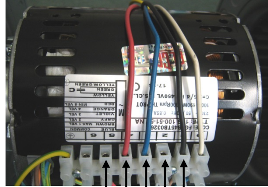
motoraftappunten: 5 4 3 2 1
